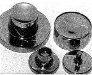
デジタルカメラ用・携帯電話用「非球面コアフランック」
